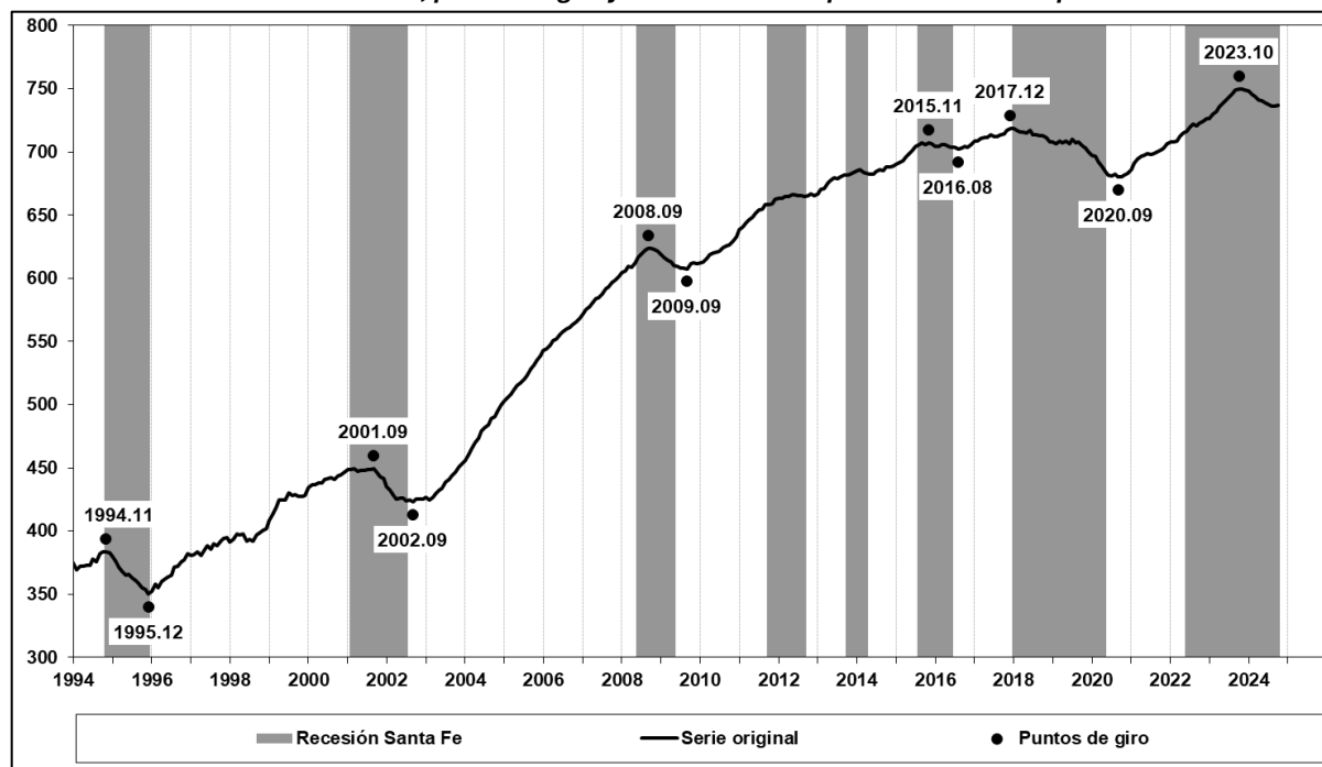
Serie N° 2: SFE-NTTA. Serie filtrada, puntos de giro y recesiones de la provincia. Miles de puestos.
