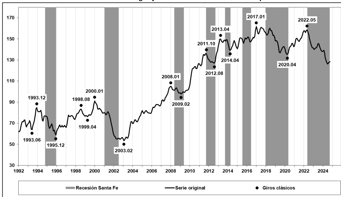
Serie N° 7: SFE-RTT. Serie filtrada. Puntos de giro y recesiones Santa Fe. Millones de pesos de 1993.
