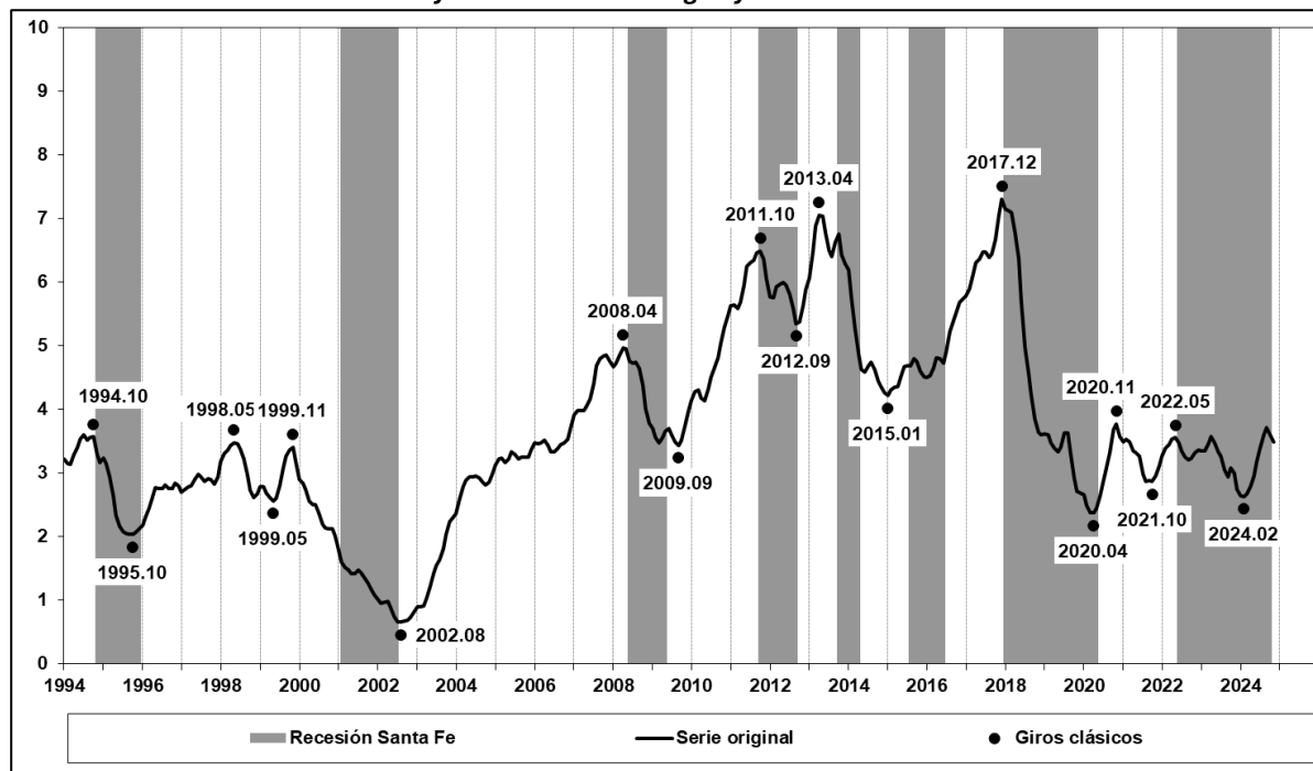
Serie N° 9: SFE-RGVN. Serie filtrada y filtro HP. Puntos de giro y recesiones Santa Fe. Miles de vehículos.
