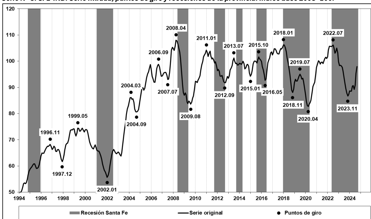
Serie N° 5: SFE-IND. Serie filtrada, puntos de giro y recesiones de la provincia. Índice base 2008=100.
