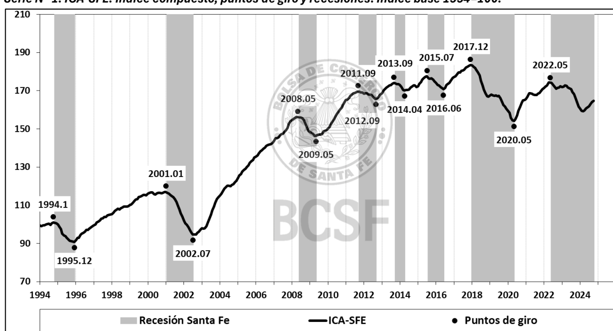
Serie N° 1: ICA-SFE. Índice compuesto, puntos de giro y recesiones. Índice base 1994=100.
