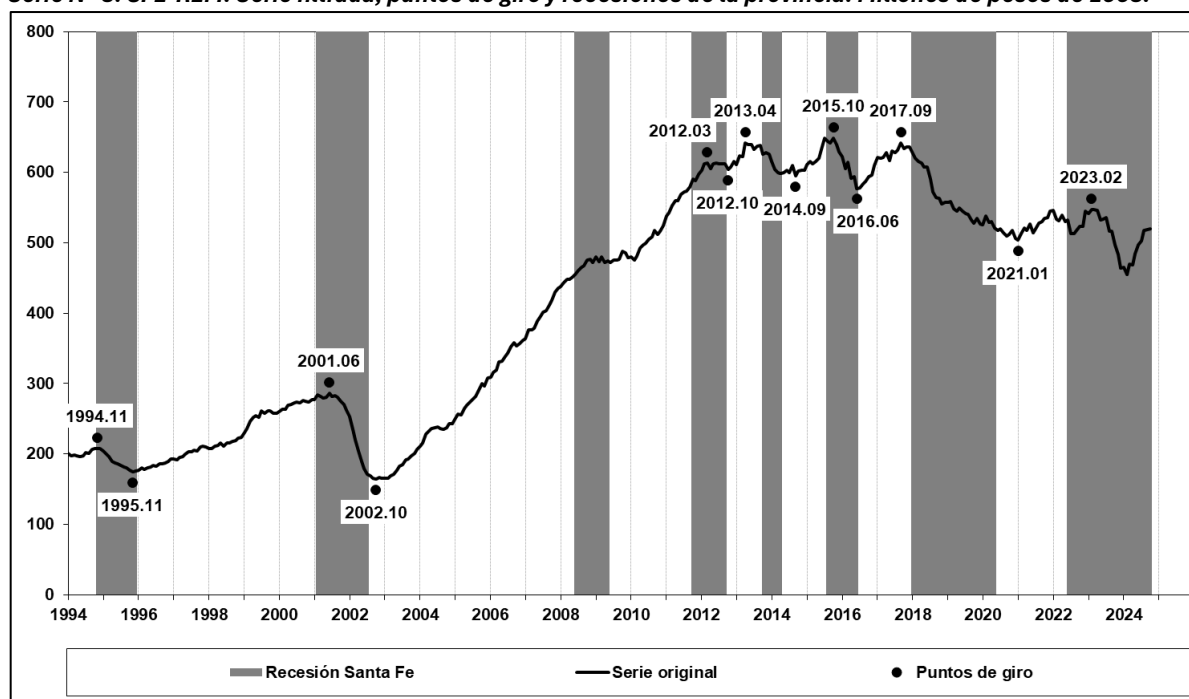
Serie N° 3: SFE-REM. Serie filtrada, puntos de giro y recesiones de la provincia. Millones de pesos de 1993.
