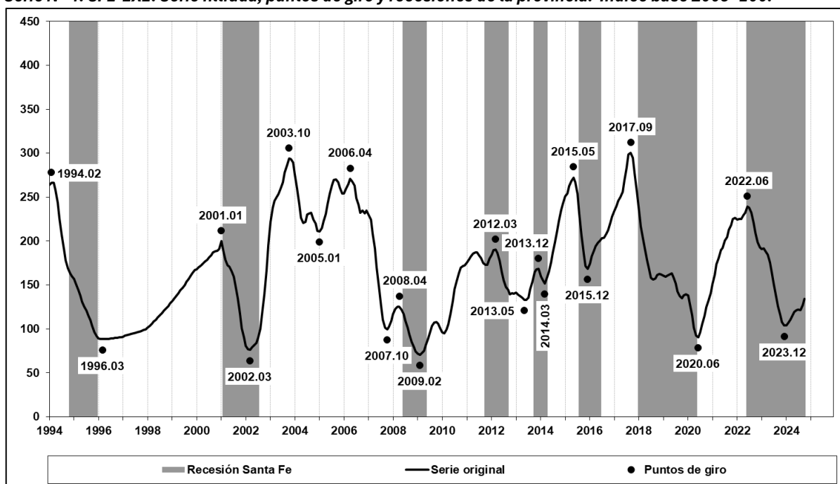
Serie N° 4: SFE-EXE. Serie filtrada, puntos de giro y recesiones de la provincia. Índice base 2009=100.
